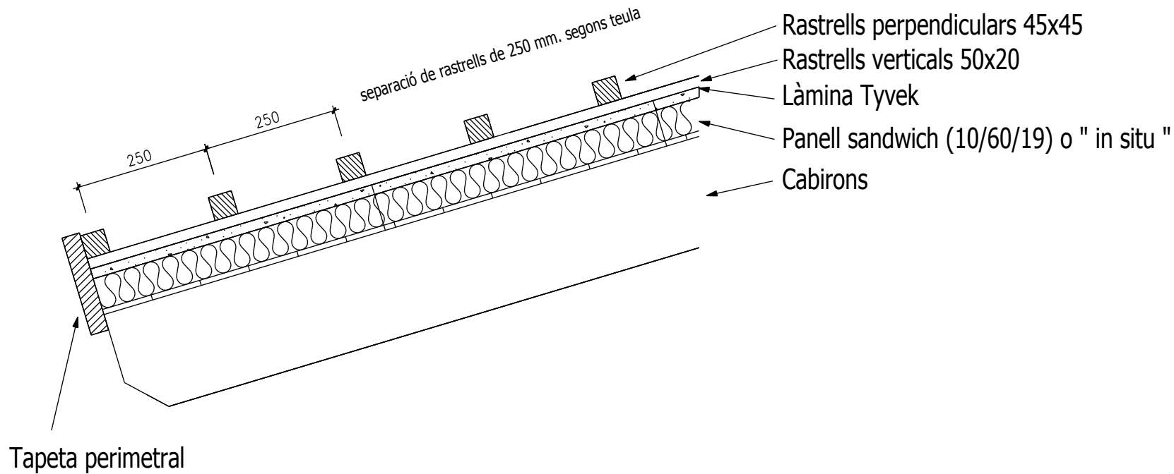
Secció lateral 1:10
