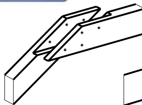
Mitja-mossa amb angle
